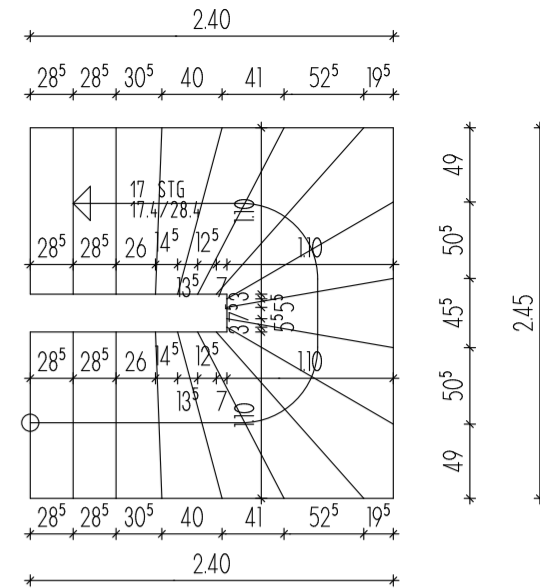
Stiege EG-DG
